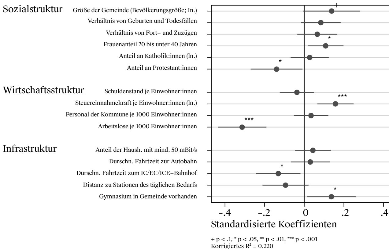
ABB. 12: REGRESSIONSMODELL FDP
