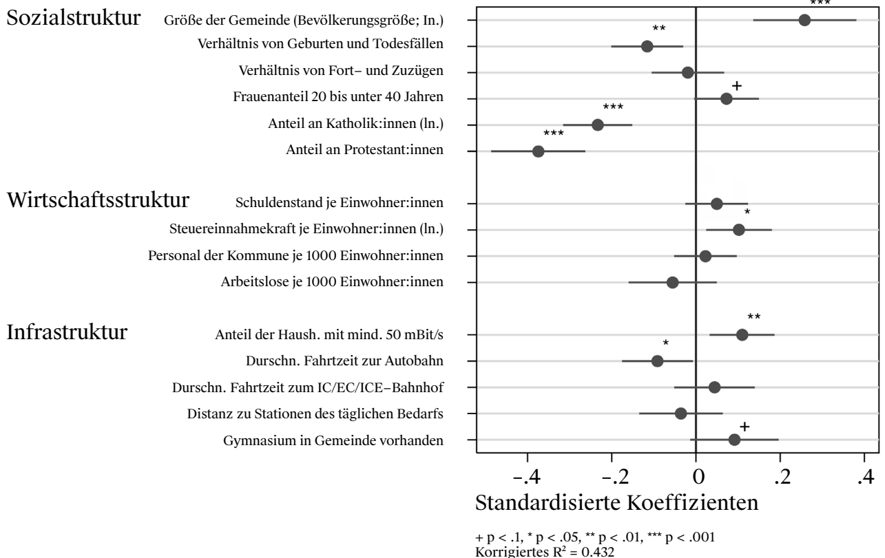
ABB. 10: REGRESSIONSMODELL SPD
