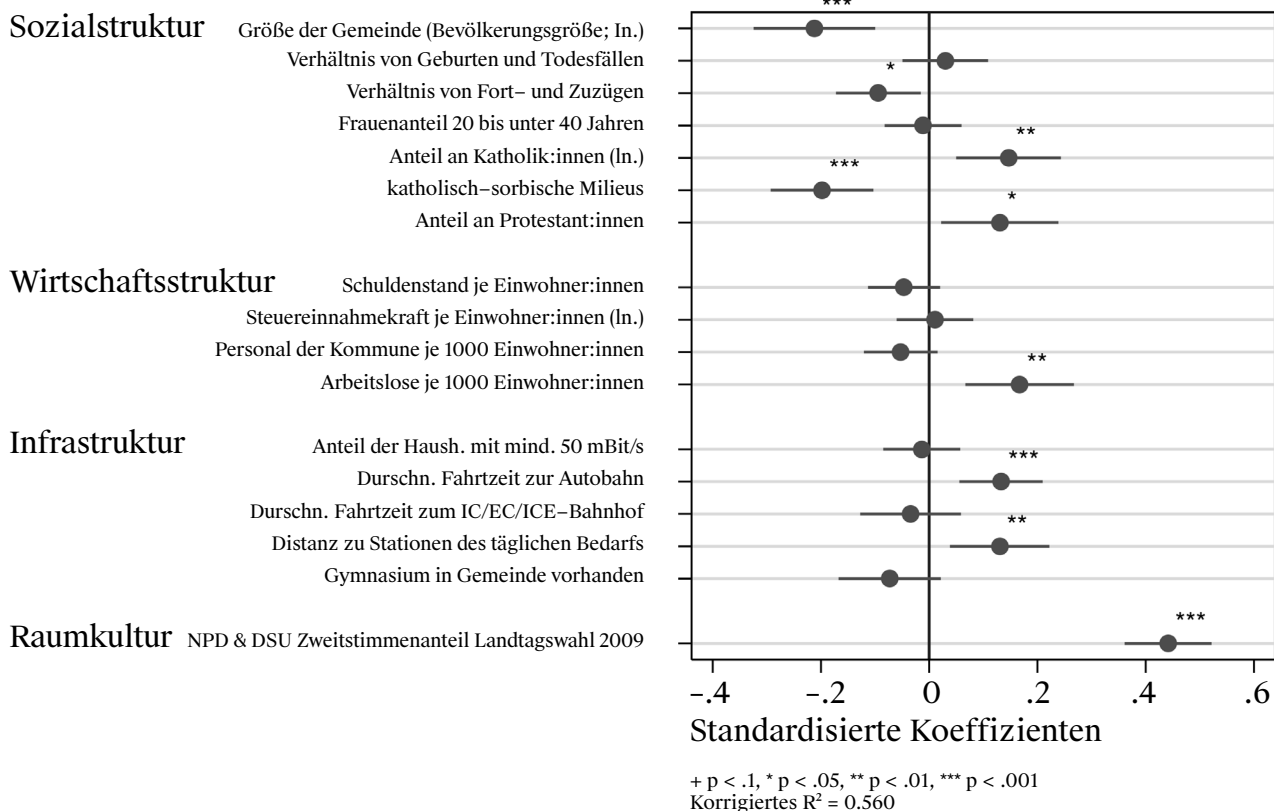
ABB. 2: REGRESSIONSMODELL AFD
