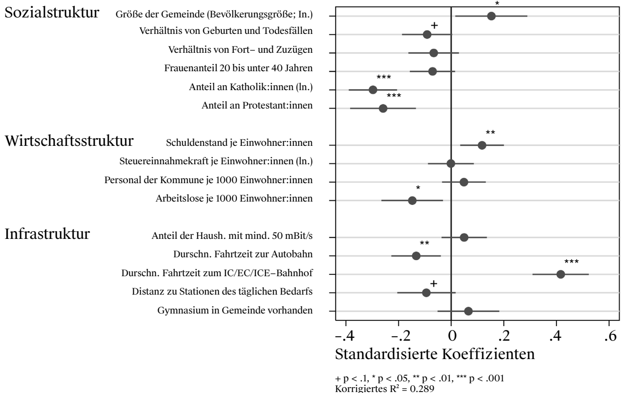
ABB. 14: REGRESSIONSMODELL BSW
