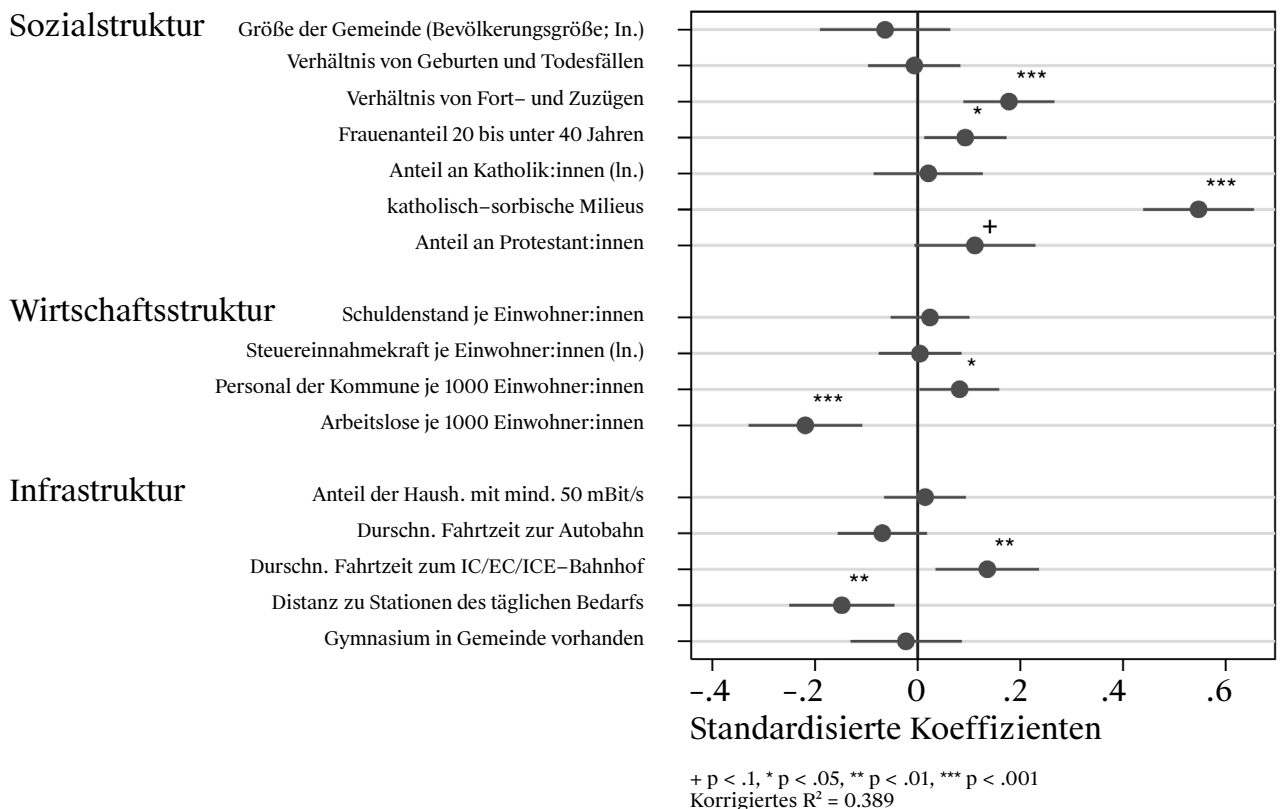
ABB. 6: REGRESSIONSMODELL CDU
